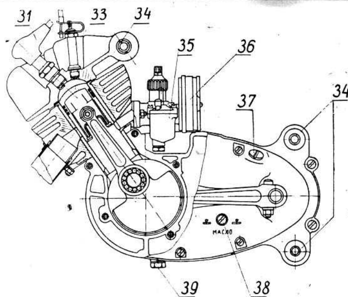
Рис. 3 — Двигатель (разрез):
